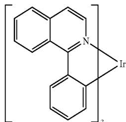
Ir(piq) 3
