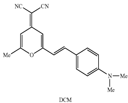
DCM
