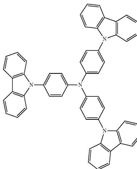
TCTA
