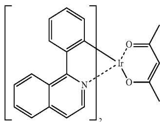
Btp 2 Ir(acac)
